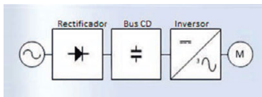
Figura 3. Diagrama en bloques de un variador típico.
