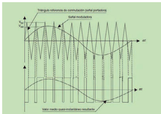
Figura 4. Esquema de operación del PWM.
