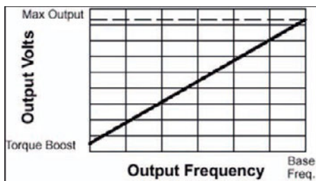
Figura 6. Curva del modo escalar.
