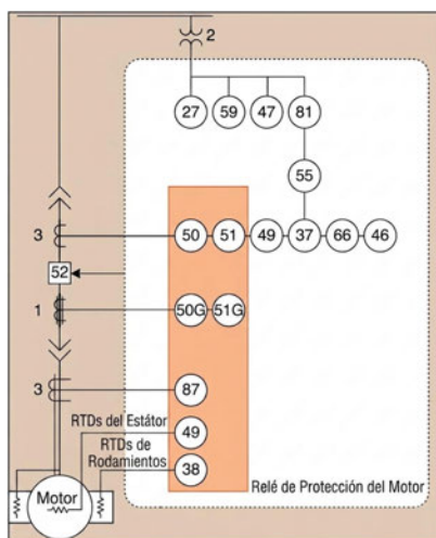
Figura 2. Diagrama unifilar de conexión de relé de protección para motor de media tensión.
