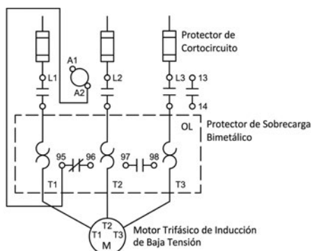
Figura 3. Diagrama de conexión de un motor trifásico (según normas norteamericanas).
