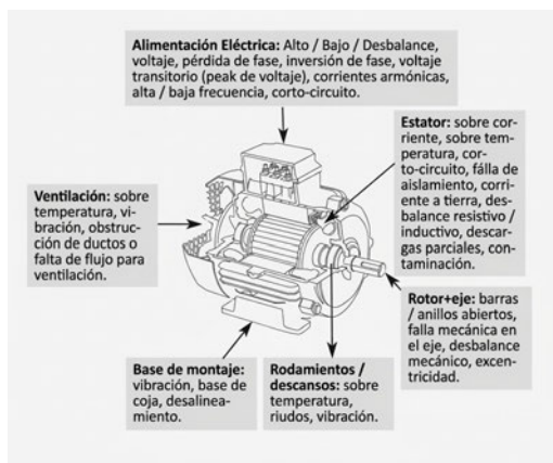
Figura 1. Zonas de protección en un motor eléctrico y causas de falla.
